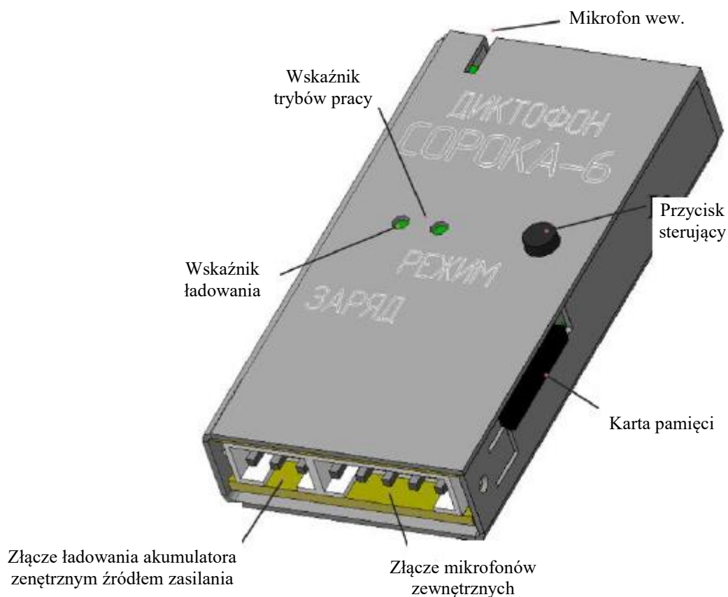
Rys. 2. Rejestrator Soroka-06E
